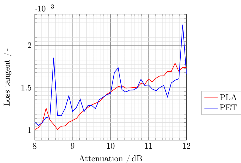
Obrázek 4-18: Výsledky extrakce ztrátového činitele materiálů Plasty Mladeč transparent PLA a PET
