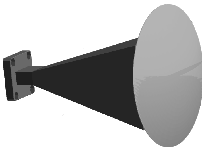
Obrázek 3-9: Výsledný model trychtýřové antény včetně čočky
