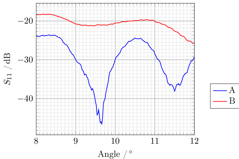
Obrázek 4-10: Naměřené impedanční přizpůsobení realizované trychtýřové antény za použití A - F-electric, B - Plasty Mladeč PET transparent + EMI 25
