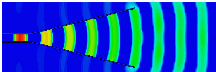
Obrázek 2-4: Princip trychtýřové antény
