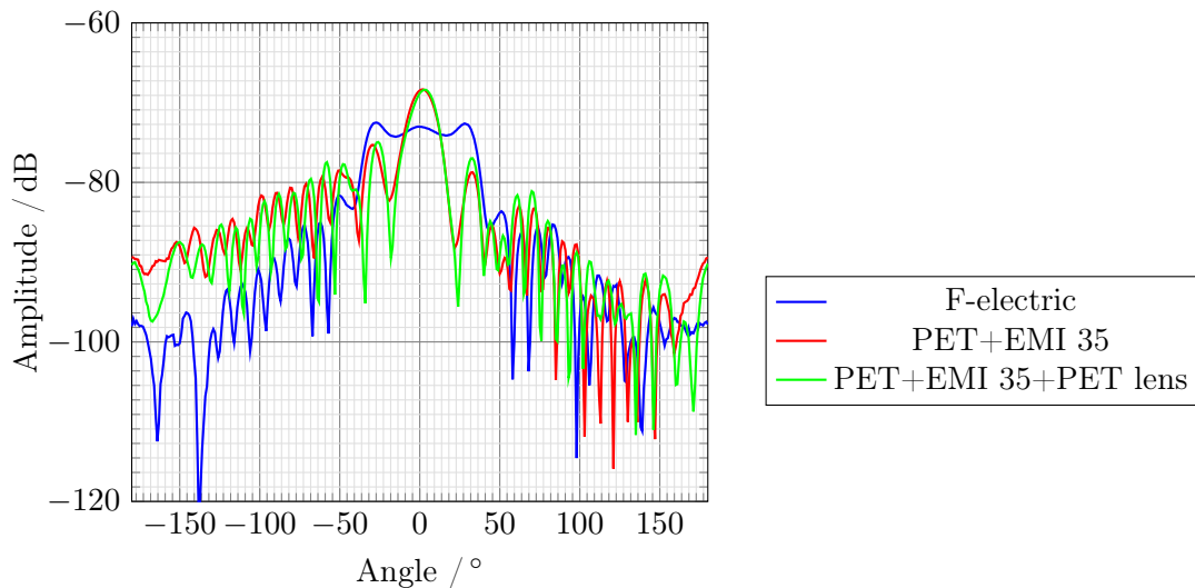
Obrázek 4-12: Naměřené vyzařovací charakteristiky realizovaných trychtýřů v H rovině
