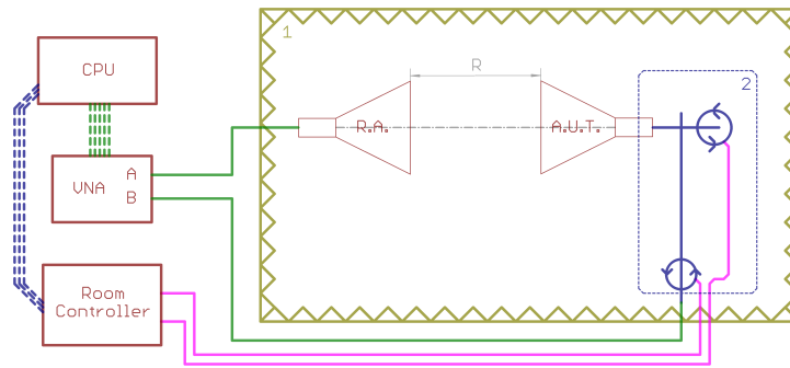
Obrázek 4-11: Zjednodušené blokové schéma měření směrové charakteristiky
