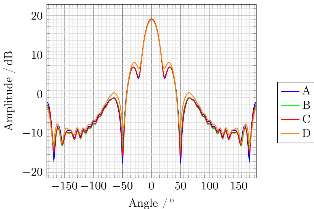
Obrázek 3-2: Řezy směrových charakteristik v E rovině, kde: A - p = 140 \text{ mm} , B - plth = 1.45 \text{ mm} , C - plth = 0.9 \text{ mm} , D - plth = 1.45 \text{ mm} ; G = 133.3 \text{ S/m}
