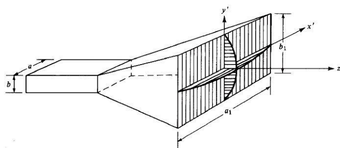
Obrázek 2-7: Pyramidální trychtýřová anténa [3]
