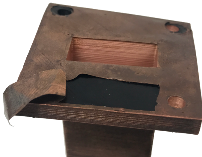
Obrázek 4-8: Nízká přilnavost k hladkým povrchům
