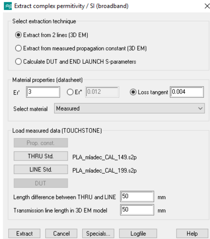
Obrázek 4-16: Náhled vhodně nakonfigurovaného uživatelského rozhraní makra v CST MW studio
