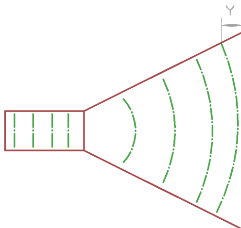
Obrázek 2-9: Znázornění fázové chyby Y
