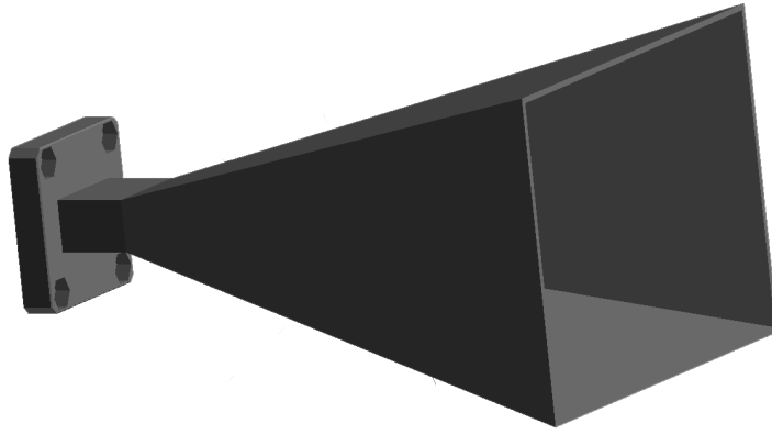
Obrázek 3-3: Výsledný model trychtýřové antény včetně příruby na vlnovod
