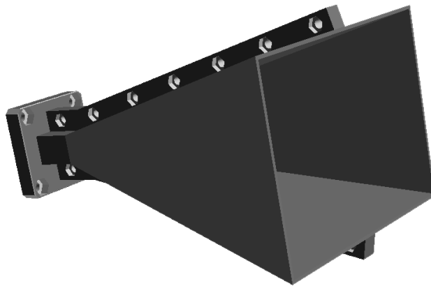
Obrázek 3-4: Výsledný model trychtýřové antény včetně příruby na vlnovod a následné sestavení
