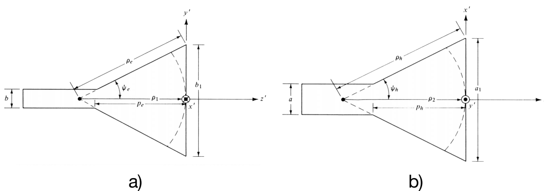
Obrázek 2-8: Pyramidální trychtýřová anténa v řezu a)E-roviny, b)H-roviny [3]
