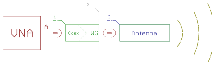
Obrázek 4-9: Blokové schéma měření impedančního přizpůsobení
