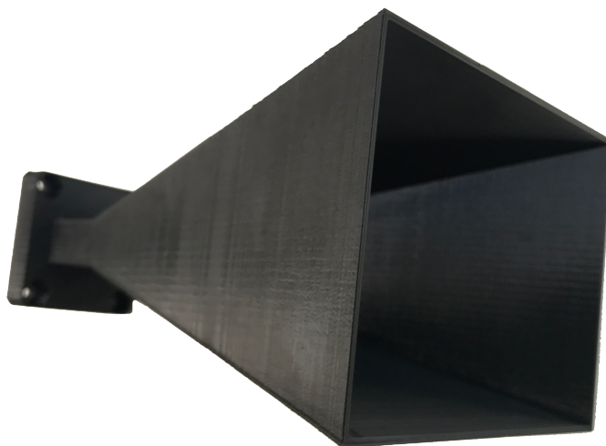
Obrázek 4-2: Výsledný model trychtýřové antény včetně příruby na vlnovod realizovaný technologií 3D tisku za použití F-electric filamentu
