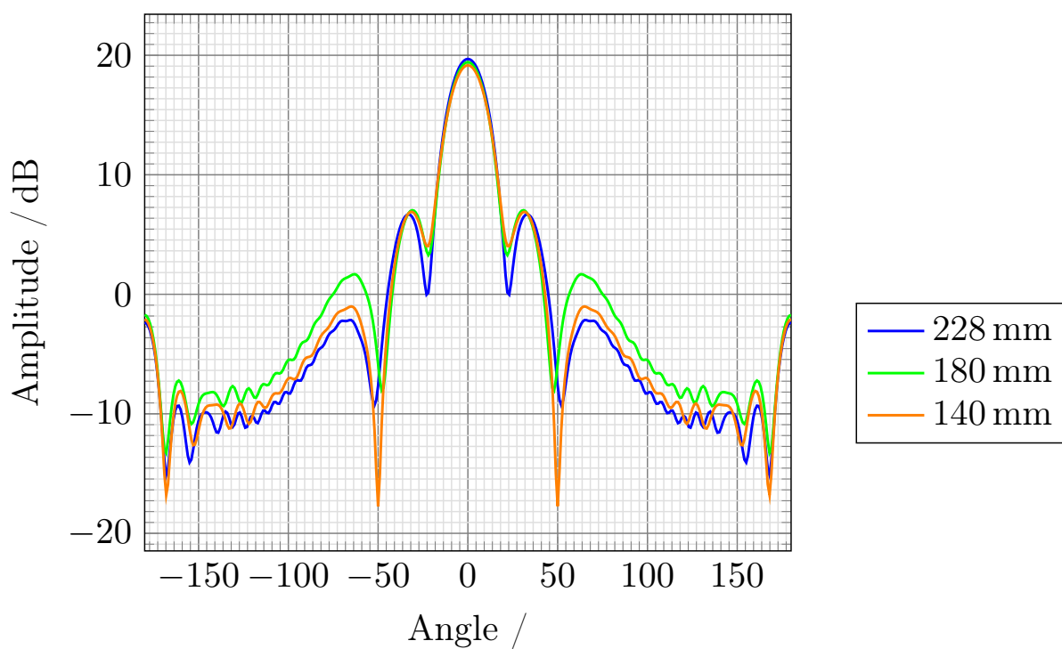
Obrázek 2-10: Řezy směrových charakteristik v E rovině pro různé délky pyramidálního trychtýře při zachování rozměrů apertury (CST MW studio simulace)
