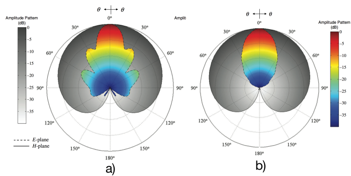
Obrázek 2-6: Porovnání směrových charakteristik trychtýřové antény s otevřením v rovině a) E , b) H [3]
