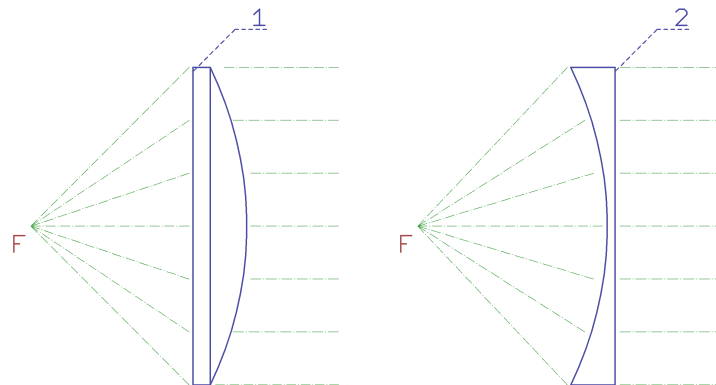
Obrázek 2-12: Typy anténních čoček. 1 - Zpomalující, 2 - Zrychlující
