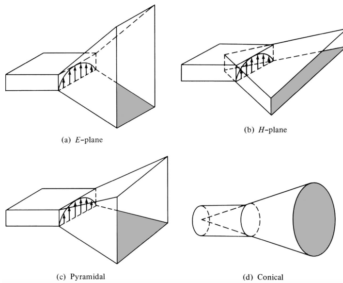
Obrázek 2-5: Typické provedení trychtýřových antén [3]
