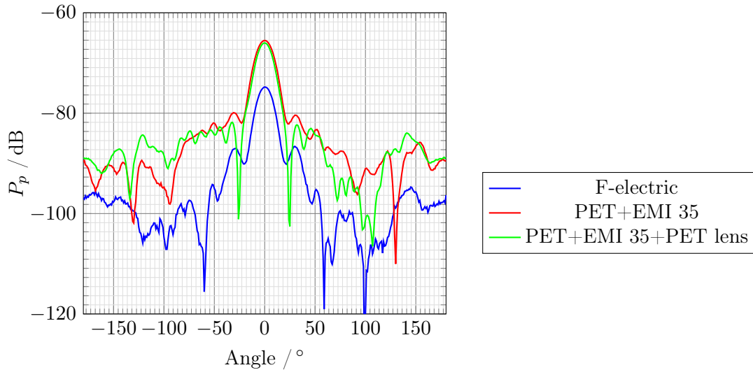
Obrázek 4-13: Naměřené vyzařovací charakteristiky realizovaných trychtýřů v E rovině
