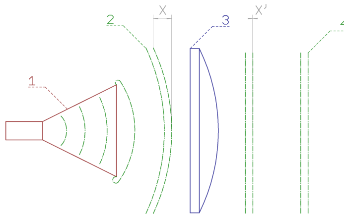
Obrázek 2-11: Princip anténní čočky
