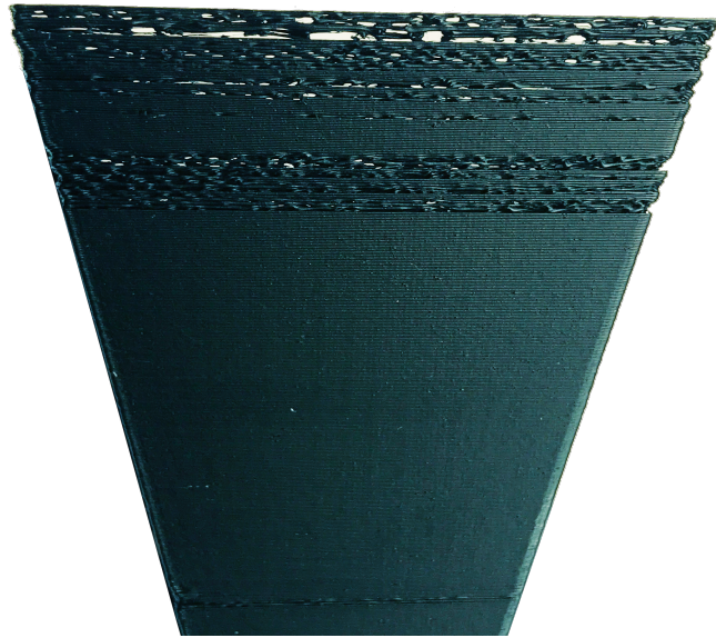
Obrázek 4-3: Důsledek ucpávání trysky v průběhu tisku modelu
