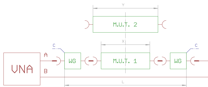
Obrázek 3-6: Blokové schéma transmisní/reflexní extrakce dielektrických parametrů
