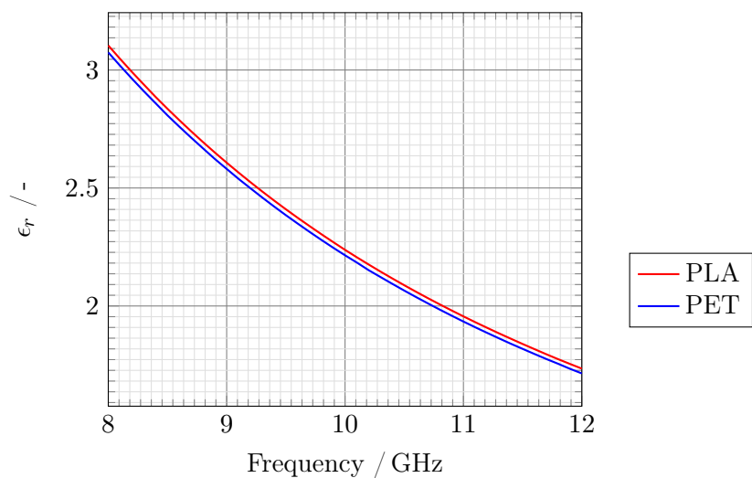
Obrázek 4-17: Výsledky extrakce komplexní permitivity materiálů Plasty Mladeč transparent PLA a PET
