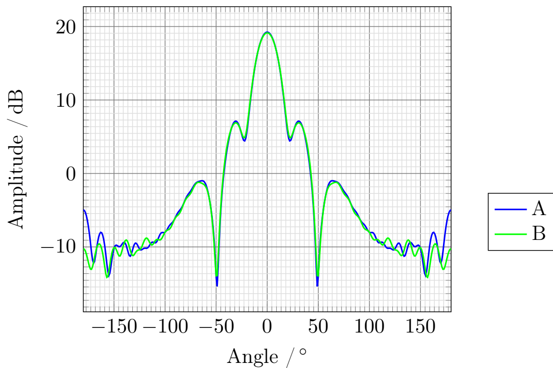
Obrázek 3-5: Řezy směrových charakteristik v E rovině, kde: A - Původní optimalizovaný trychtýř, B - Trychtýř s přírubami na sestavení
